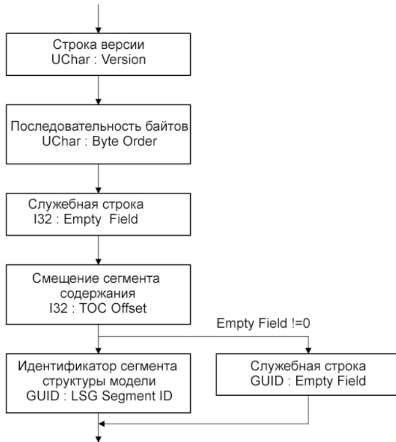
Рисунок 3 — Данные сегмента заголовка файла
