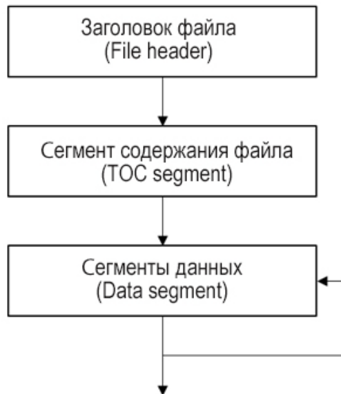
Рисунок 1 — Структура файла JT
